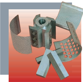
режущий ротор и вставные сита
