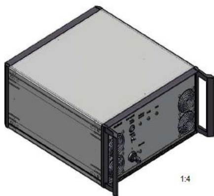
Отдельно-стоящий блок управления Длина: 375 мм; Ширина: 356 мм; Высота: 184 мм (все размеры в мм)
